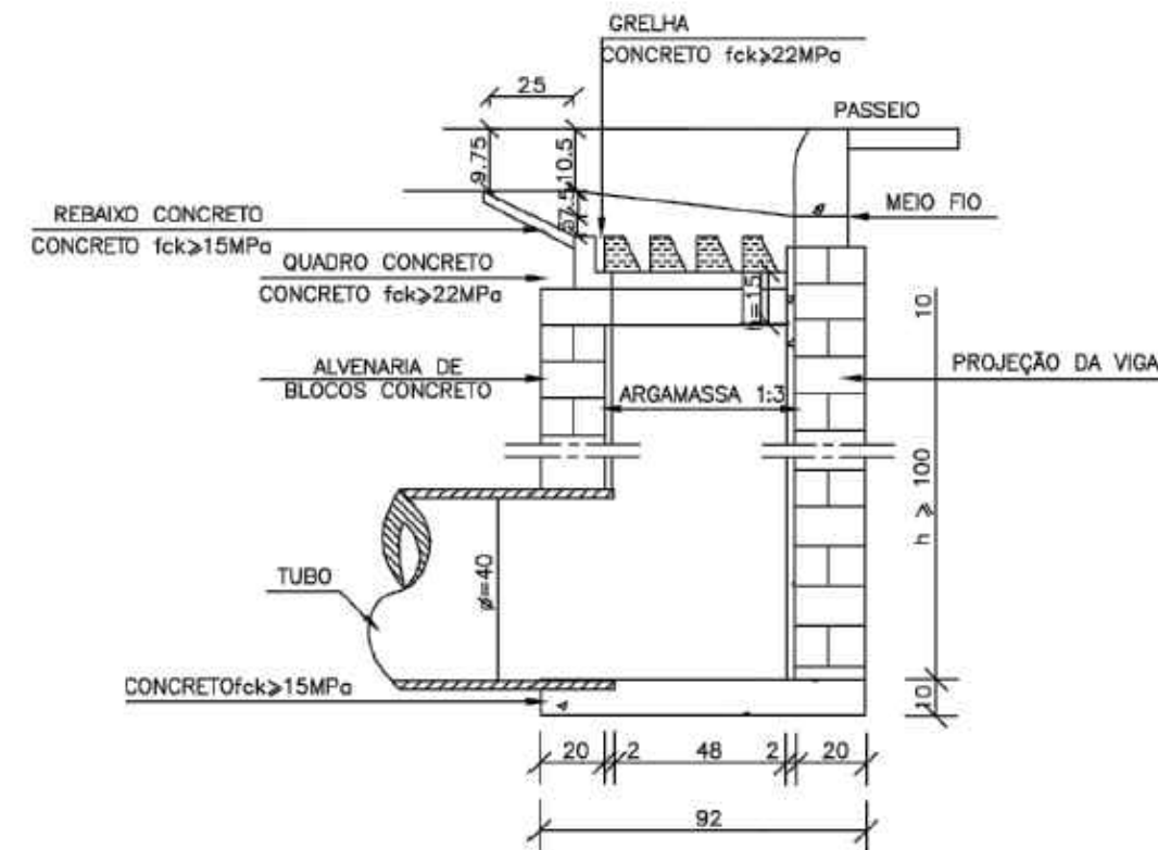
CORTE BB'
