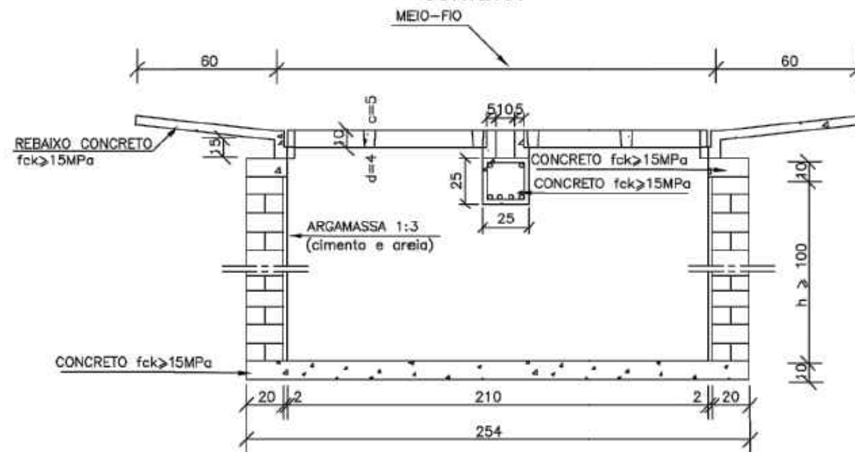
CORTE AA'
