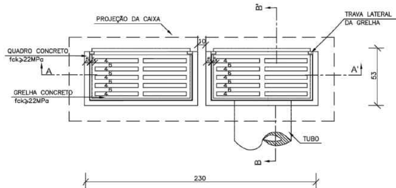
PLANTA
