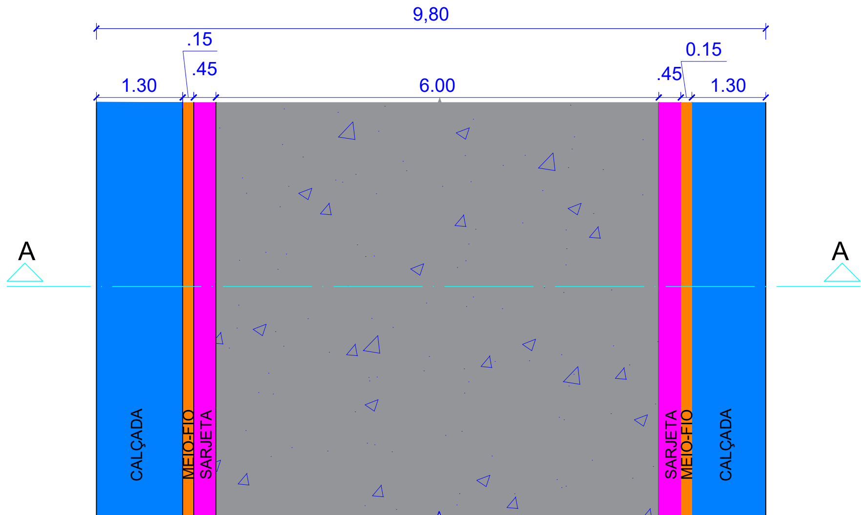
PLANTA BAIXA - PAVIMENTAÇÃO EM ASFALTO COM MEIO-FIO, SARJETA E CALÇADA - 3,00m ESC:1/50
