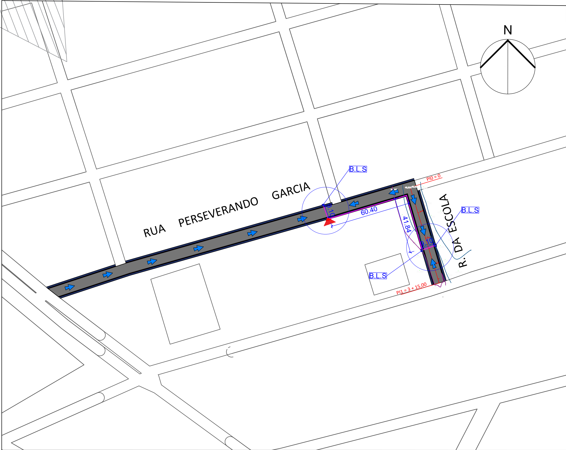
DRENAGEM - RUA PERSEVERANDO GARCIA / RUA DA ESCOLA ESC: 1/500
