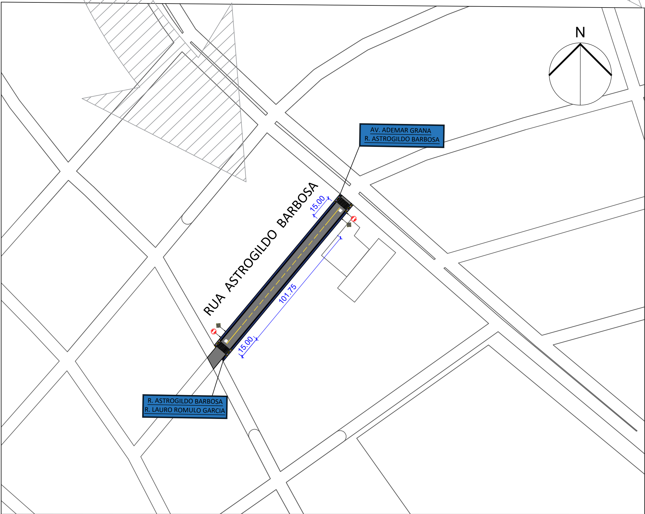
SINAL. E ACESS. - RUA ASTROGILDO BARBOSA ESC: 1/1500
