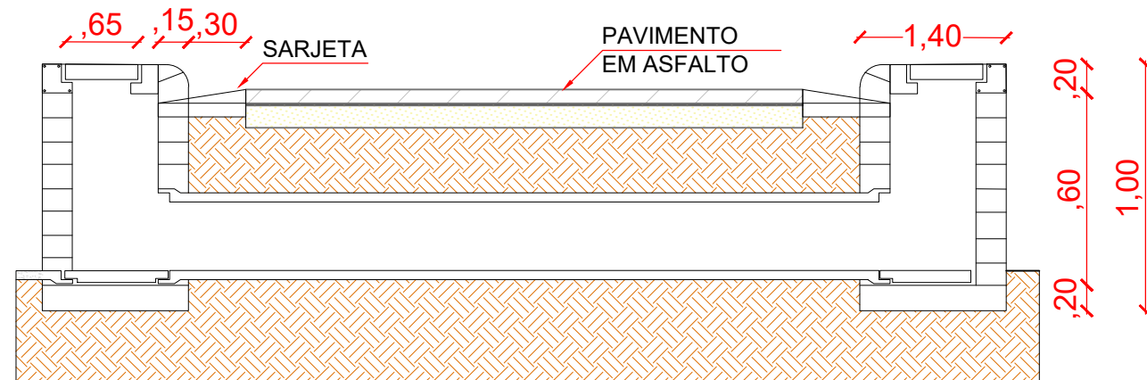
CORTE AA' - BOCA DE LOBO ESC.: 1/100
