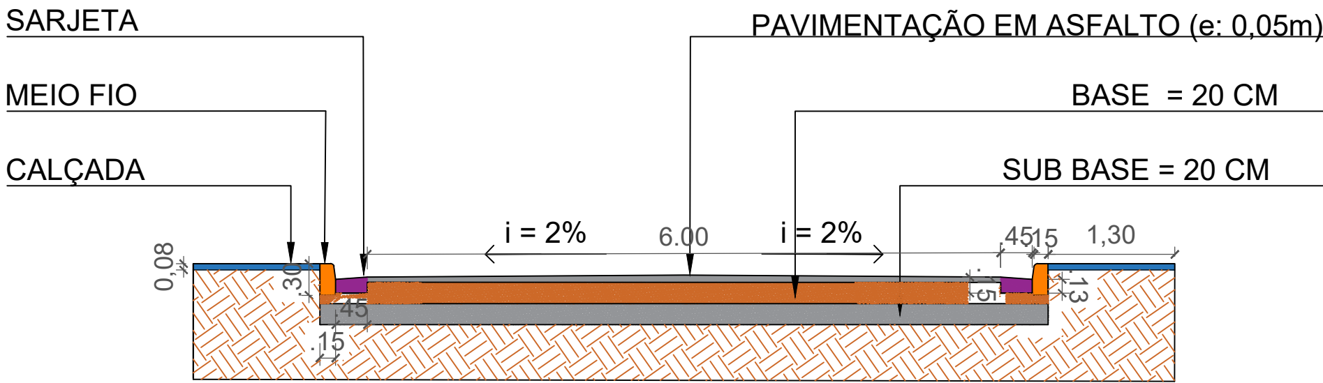
CORTE AA' - PAVIMENTAÇÃO ASFÁLTICA COM CALÇADA, MEIO-FIO/SARJETA (MFC-03)
