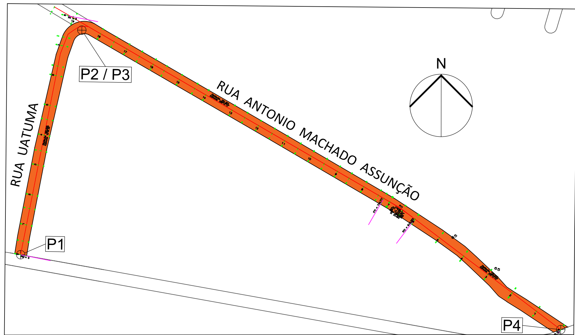
SIT. E LOCAÇÃO - RUA UATUMA / RUA ANTONIO MACHADO ASSUNÇÃO (RETIRADA) ESC: 1/1500
