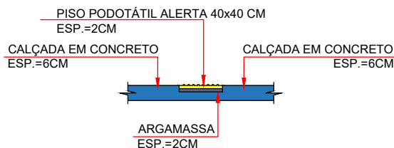
INSTALAÇÃO - PISO TÁTIL ESC.: 1/25
