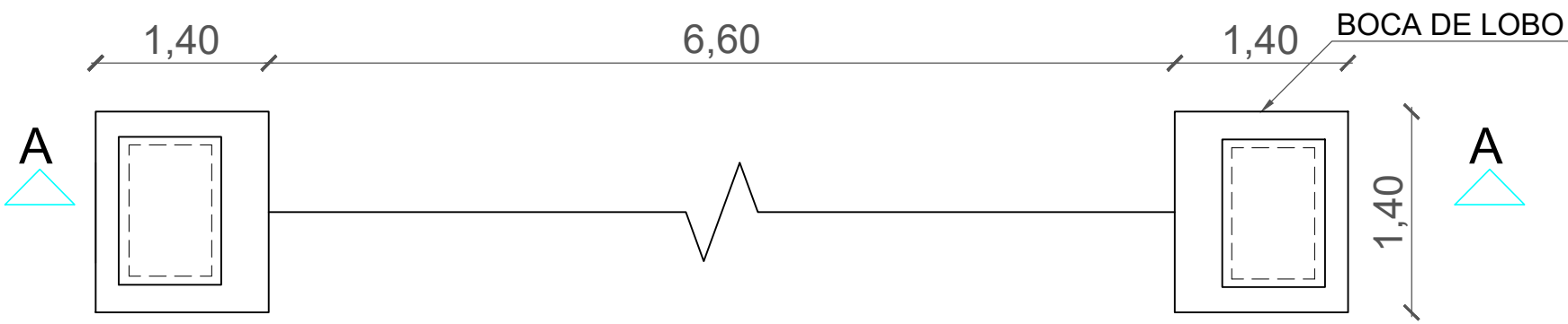
PLANTA BAIXA - BOCA DE LOBO ESC.: 1/100
