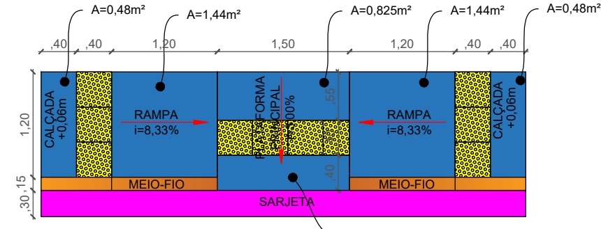
RAMPA - PLANTA BAIXA ÁREA DE PINTURA TOTAL: 5,265m² 08 UNIDADES ESC.: 1/50
