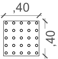
DETALHE - PISO TÁTIL ESC.: 1/25
