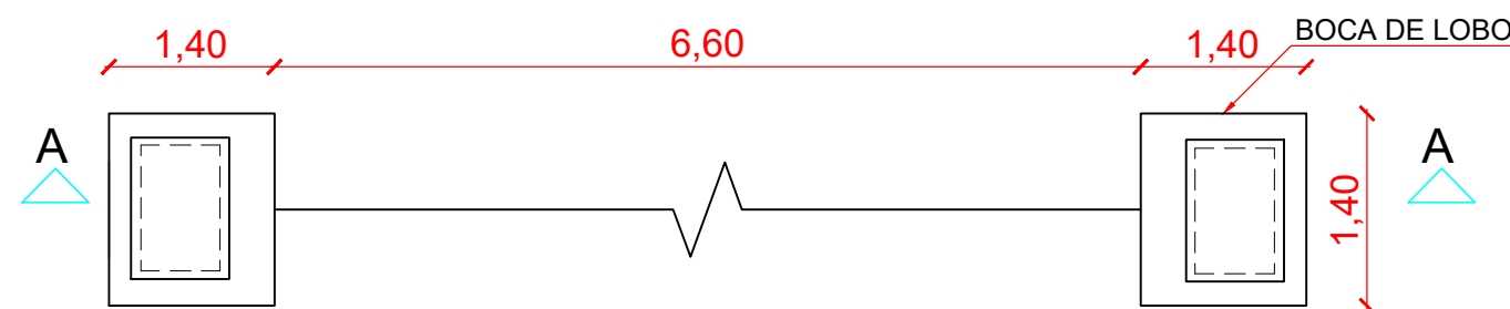
PLANTA BAIXA - BOCA DE LOBO ESC.: 1/100
