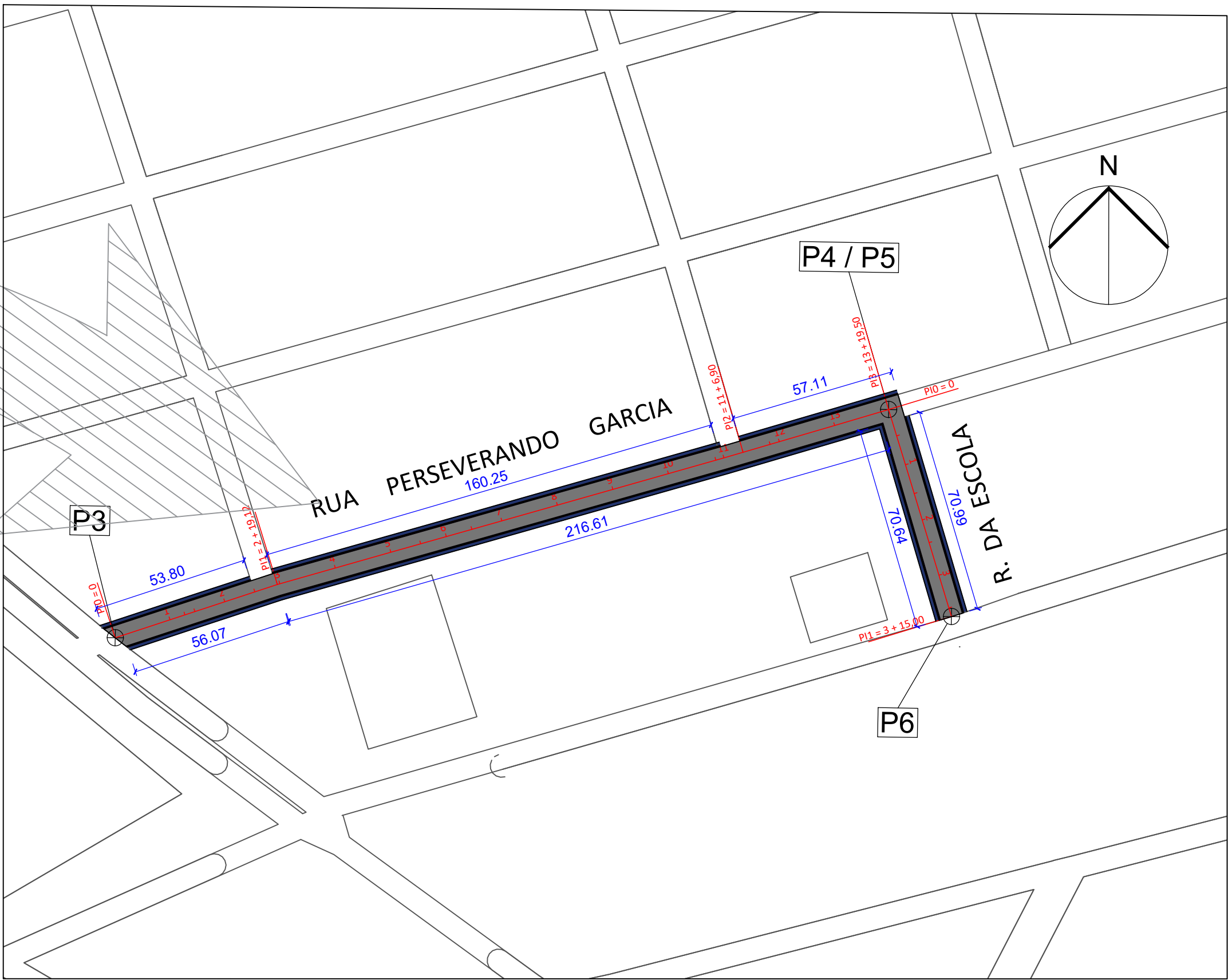
PAVIMENTAÇÃO - RUA PERSEVERANDO GARCIA / RUA DA ESCOLA ESC: 1/500
