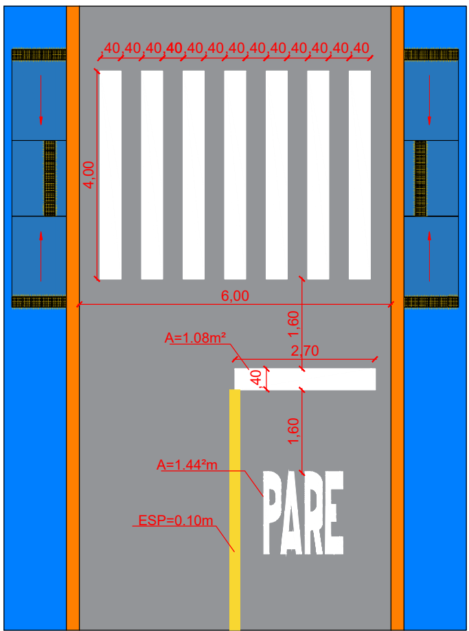
DETALHE - FAIXA DE PEDESTRES "TIPO ZEBRADA" ESC.: 1/100
