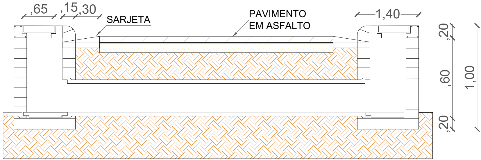
CORTE AA' - BOCA DE LOBO ESC.: 1/100
