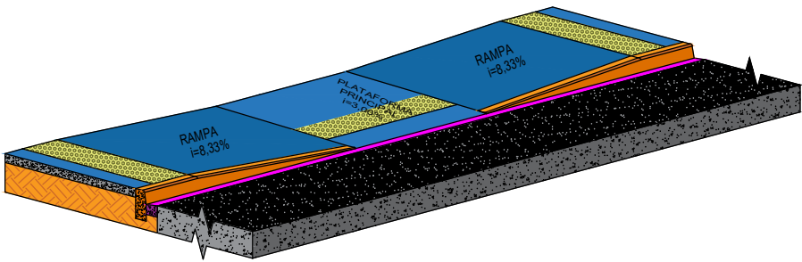
RAMPA - PERSPECTIVA ÁREA DE PINTURA TOTAL: 5,265m² 08 UNIDADES ESC.: 1/50
