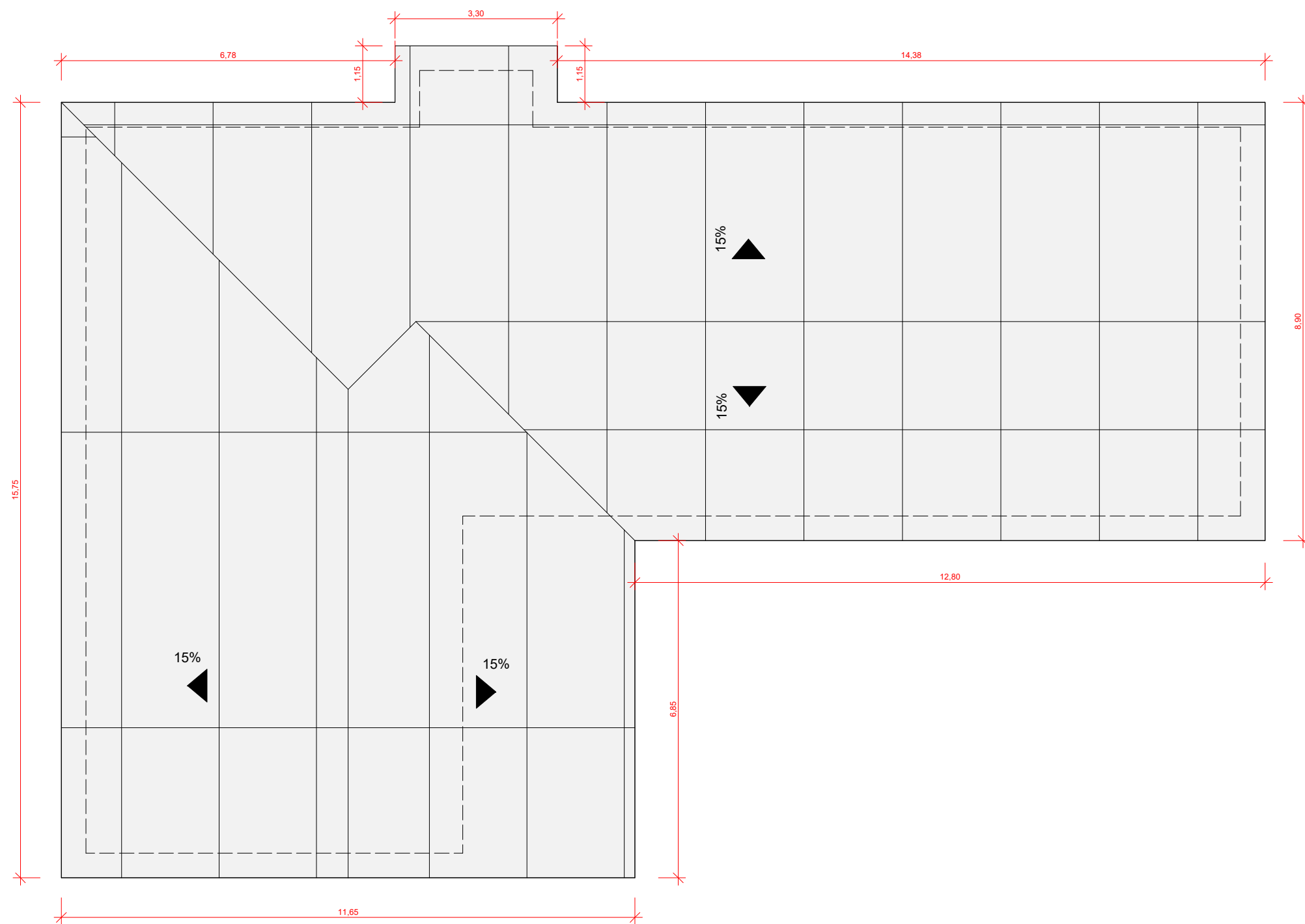
2 COBERUTA ESCALA 1 : 100
