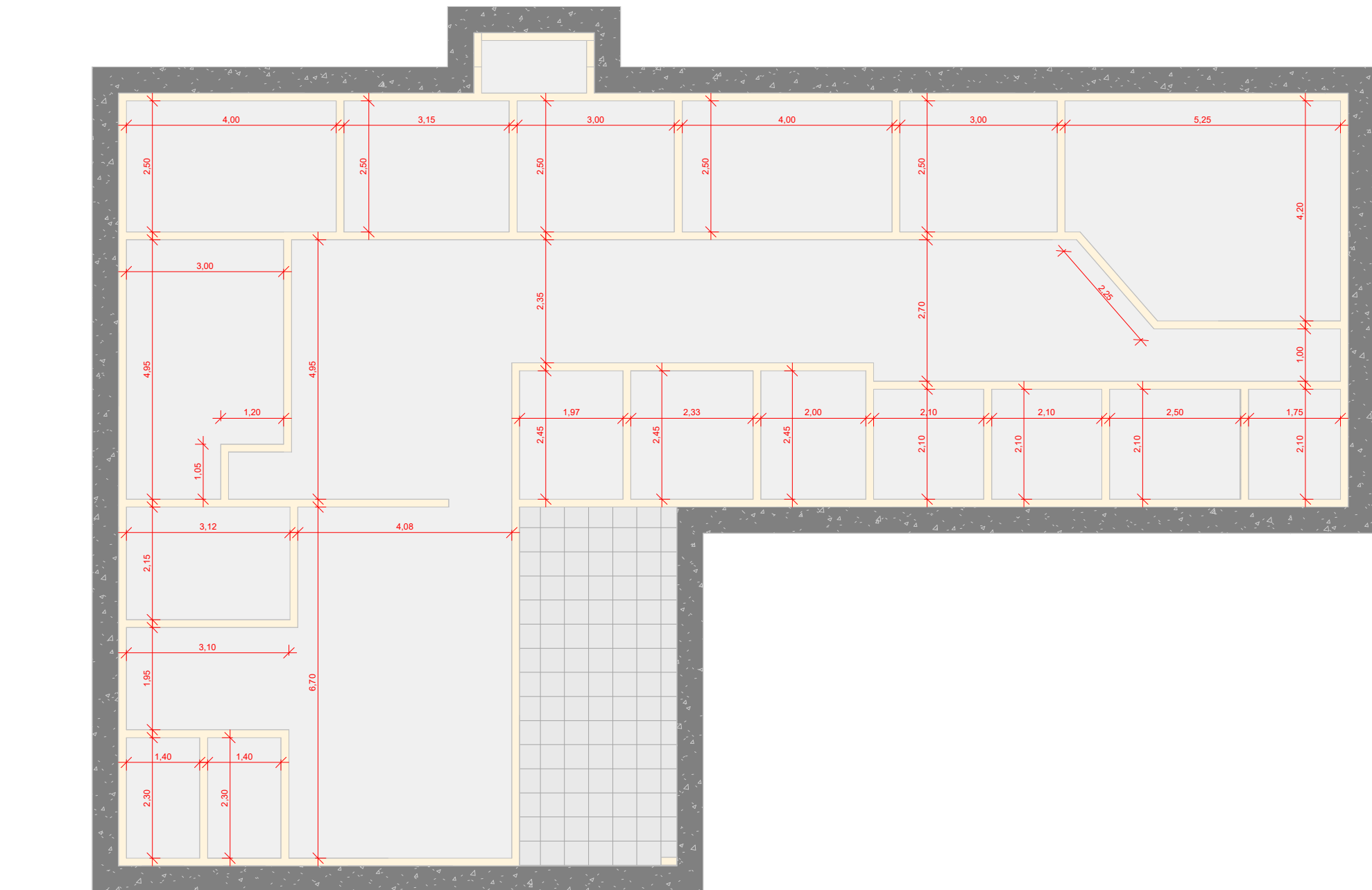
3 FORRO ESCALA 1 : 100
